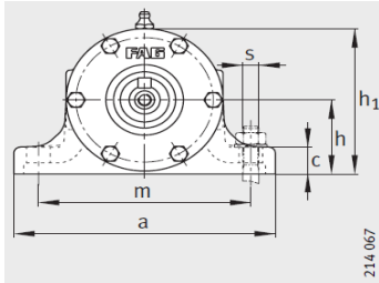
横截面 设计类型 A、B, 第 1431 页, 设计类型 C、D, 第 1433 页
